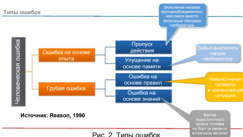
Рис. 2. Типы ошибок
